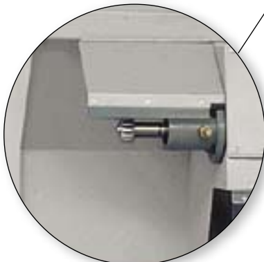
Leistenfräsanlage / last milling system
